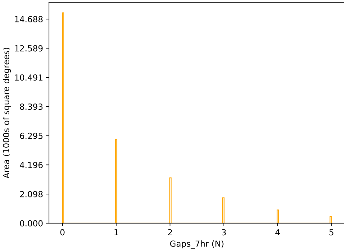
weather_cloudso20v3.4_10yrs r band: Gaps_7hr
