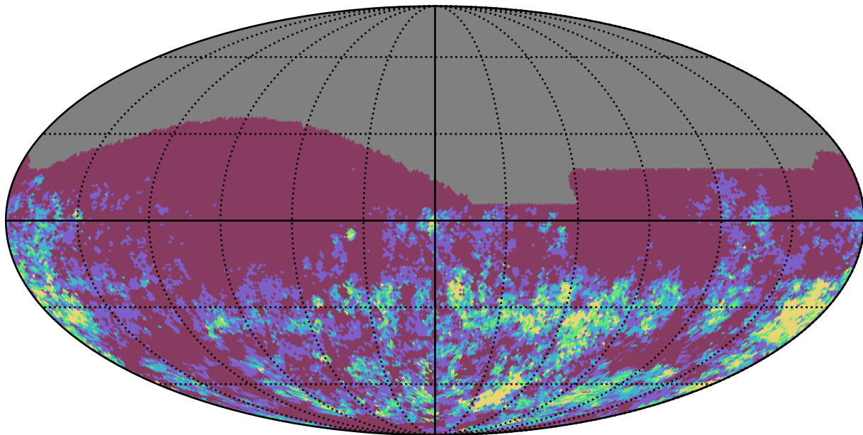
weather_cloudso20v3.4_10yrs i band: Gaps_7hr
