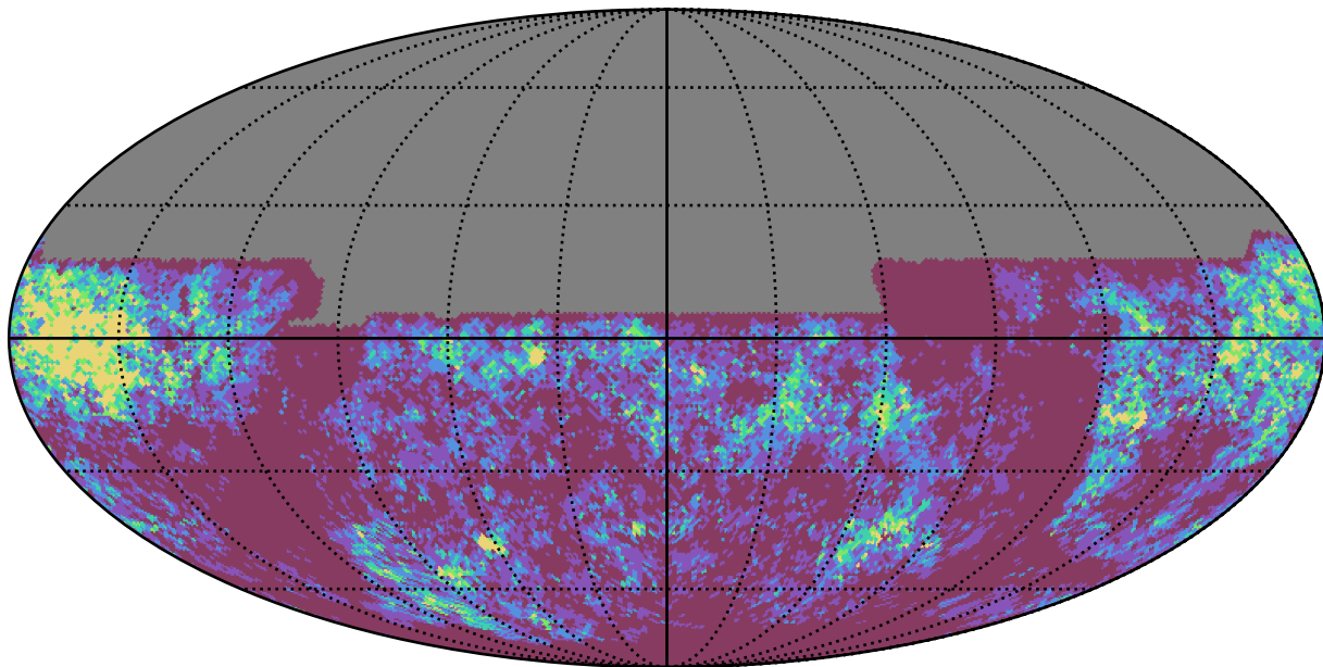
weather_cloudso20v3.4_10yrs y band: Gaps_3hr
