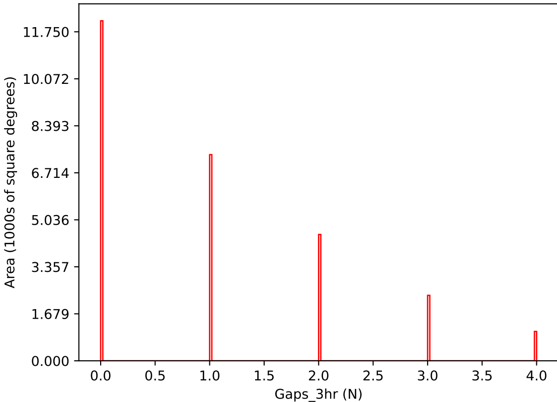
weather_cloudso20v3.4_10yrs i band: Gaps_3hr
