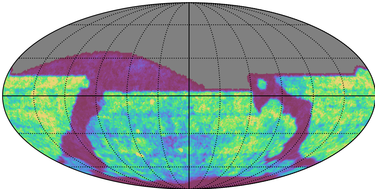
weather_cloudso20v3.4_10yrs r band: Gaps_24hr
