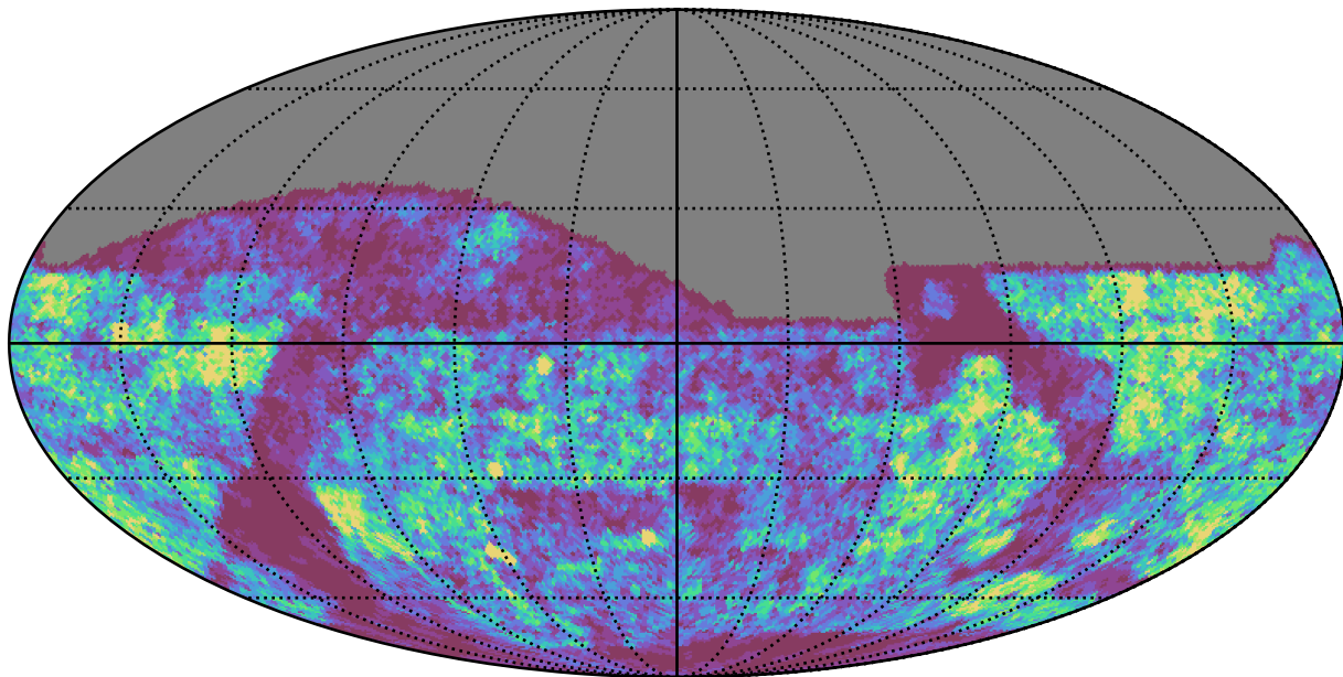
weather_cloudso20v3.4_10yrs g band: Gaps_24hr
