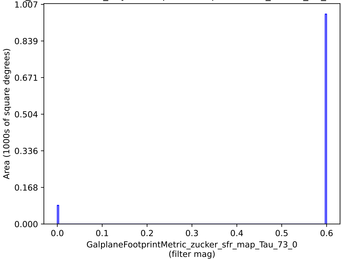
weather_cloudso20v3.4_10yrs : GalplaneFootprintMetric_zucker_sfr_map_Tau_73_0
