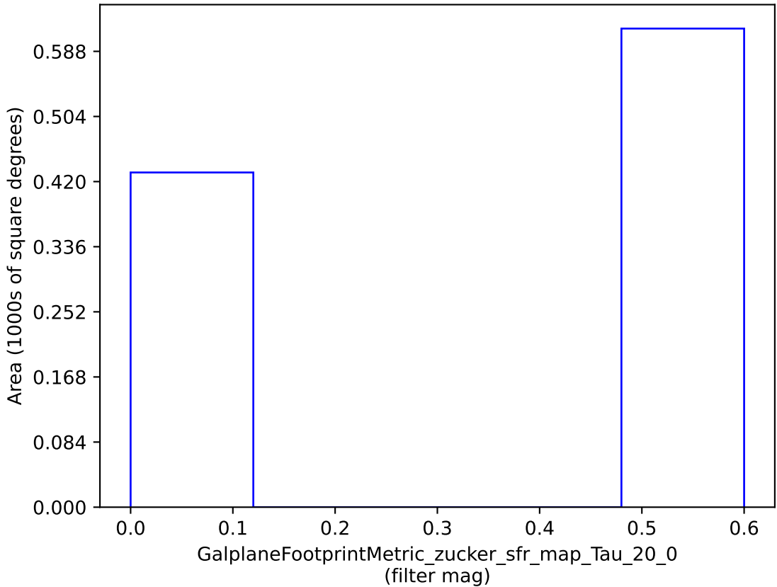
weather_cloudso20v3.4_10yrs : GalplaneFootprintMetric_zucker_sfr_map_Tau_20_0
