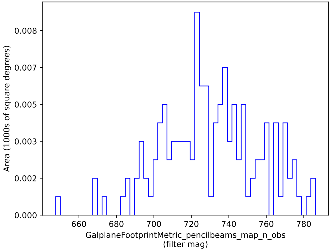
weather_cloudso20v3.4_10yrs : GalplaneFootprintMetric_pencilbeams_map_n_obs
