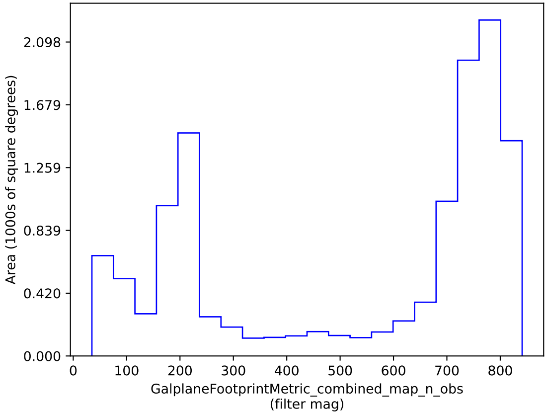
weather_cloudso20v3.4_10yrs : GalplaneFootprintMetric_combined_map_n_obs
