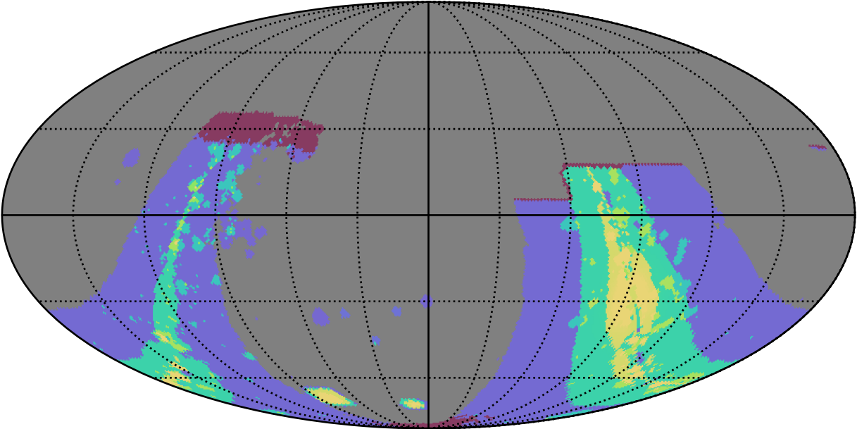
weather_cloudso20v3.4_10yrs : GalplaneFootprintMetric_combined_map_Tau_73_0
