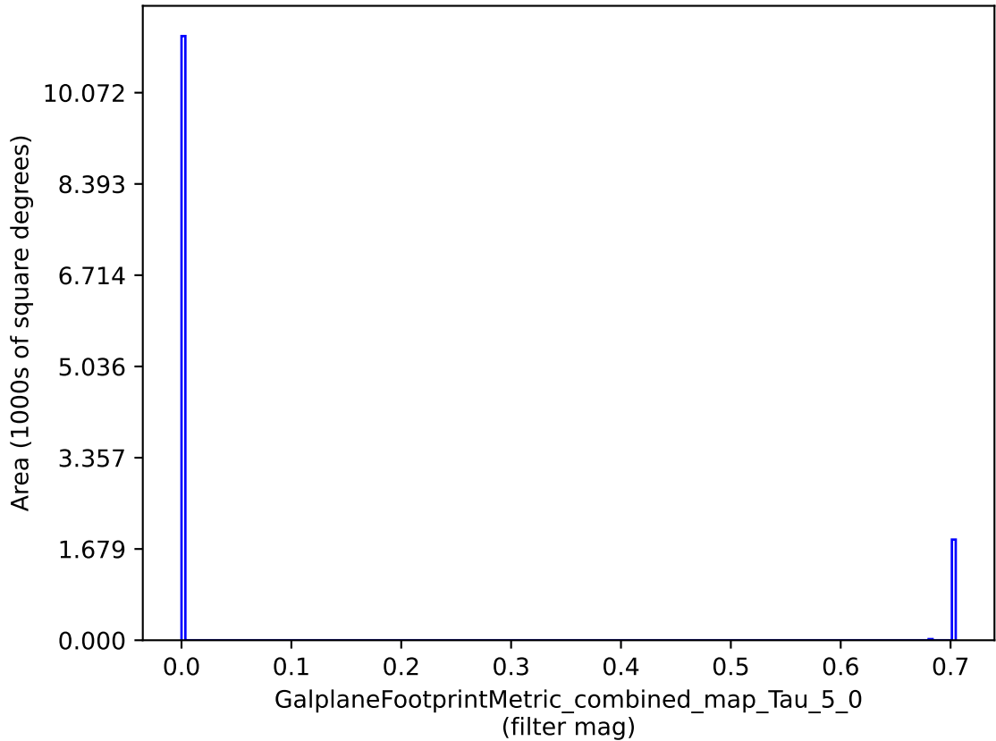
weather_cloudso20v3.4_10yrs : GalplaneFootprintMetric_combined_map_Tau_5_0
