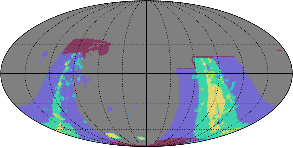
weather_cloudso20v3.4_10yrs : GalplaneFootprintMetric_combined_map_Tau_46_5
