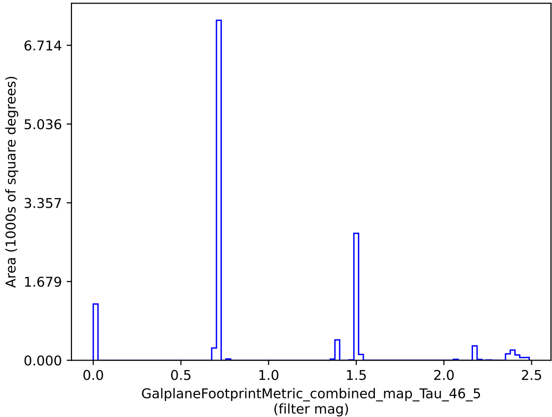
weather_cloudso20v3.4_10yrs : GalplaneFootprintMetric_combined_map_Tau_46_5
