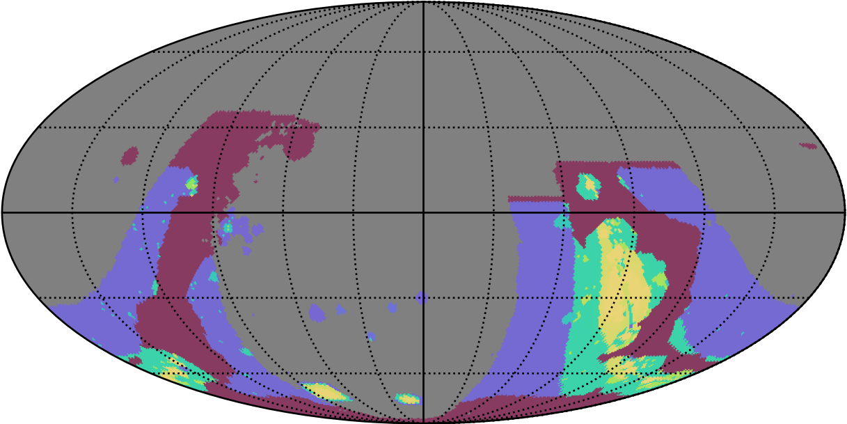
weather_cloudso20v3.4_10yrs : GalplaneFootprintMetric_combined_map_Tau_11_0
