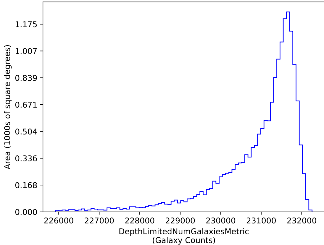
weather_cloudso20v3.4_10yrs i band galaxies non-DD: DepthLimitedNumGalaxiesMetric
