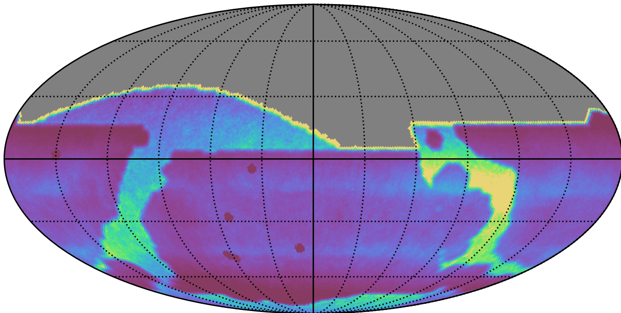
weather_cloudso20v3.4_10yrs : DCRprecision
