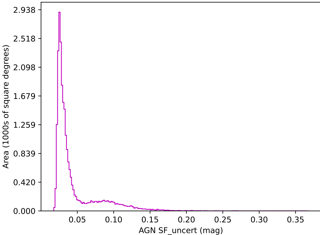
weather_cloudso20v3.4_10yrs z band: AGN SF_uncert
