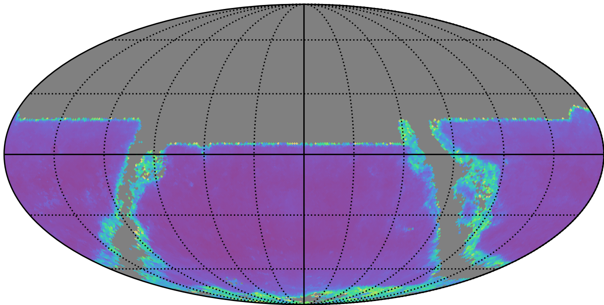
weather_cloudso20v3.4_10yrs y band: AGN SF_uncert
