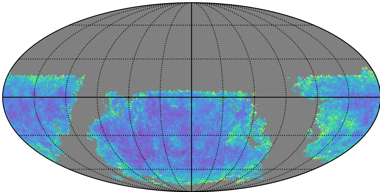
weather_cloudso20v3.4_10yrs u band: AGN SF_uncert
