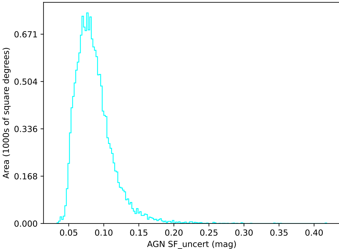
weather_cloudso20v3.4_10yrs u band: AGN SF_uncert
