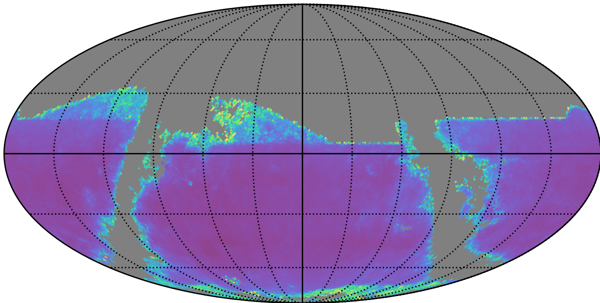
weather_cloudso20v3.4_10yrs r band: AGN SF_uncert
