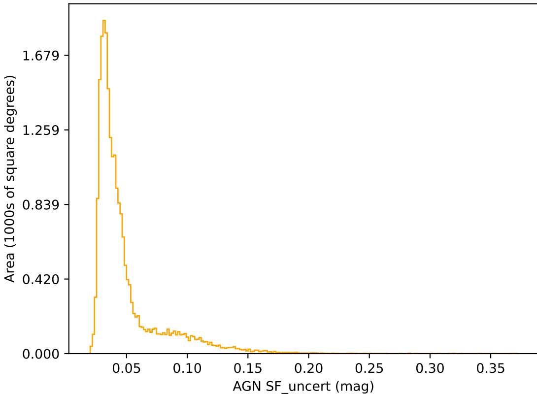
weather_cloudso20v3.4_10yrs r band: AGN SF_uncert
