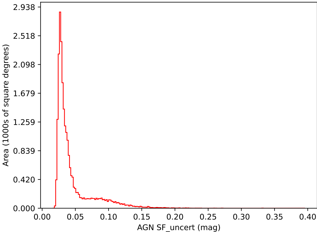
weather_cloudso20v3.4_10yrs i band: AGN SF_uncert
