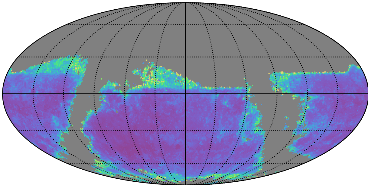
weather_cloudso20v3.4_10yrs g band: AGN SF_uncert
