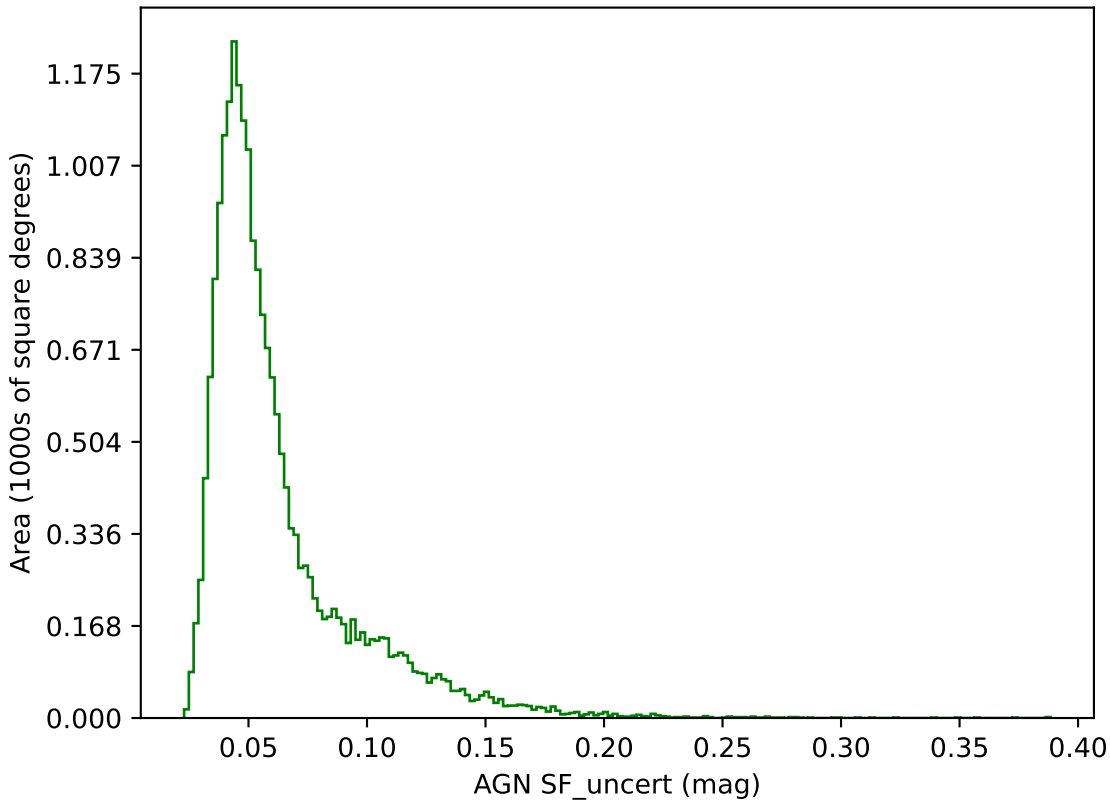
weather_cloudso20v3.4_10yrs g band: AGN SF_uncert
