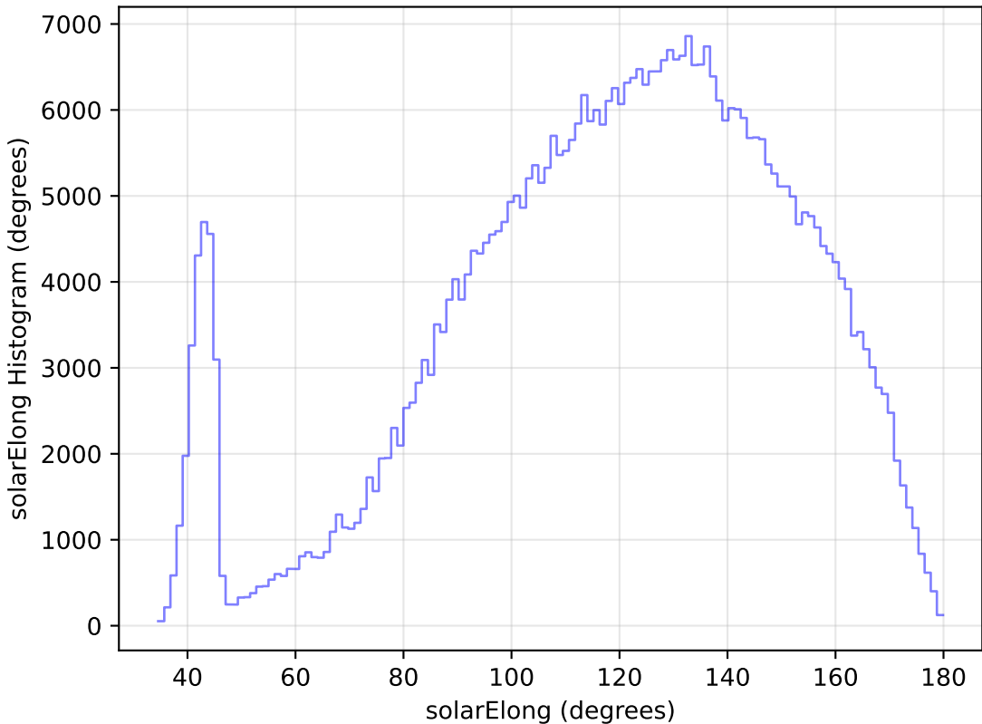
weather_cloudso20v3.4_10yrs WFD z band: solarElong Histogram
