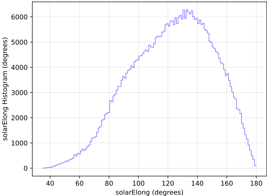
weather_cloudso20v3.4_10yrs WFD y band: solarElong Histogram
