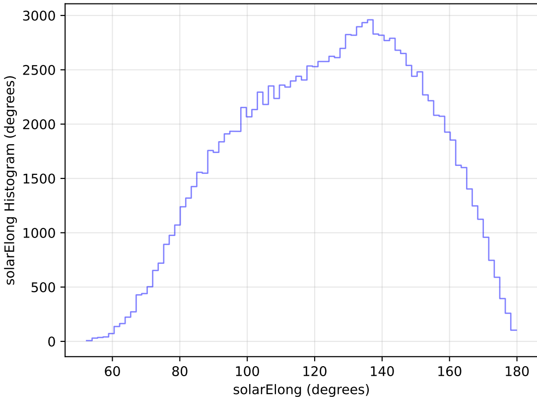
weather_cloudso20v3.4_10yrs WFD u band: solarElong Histogram
