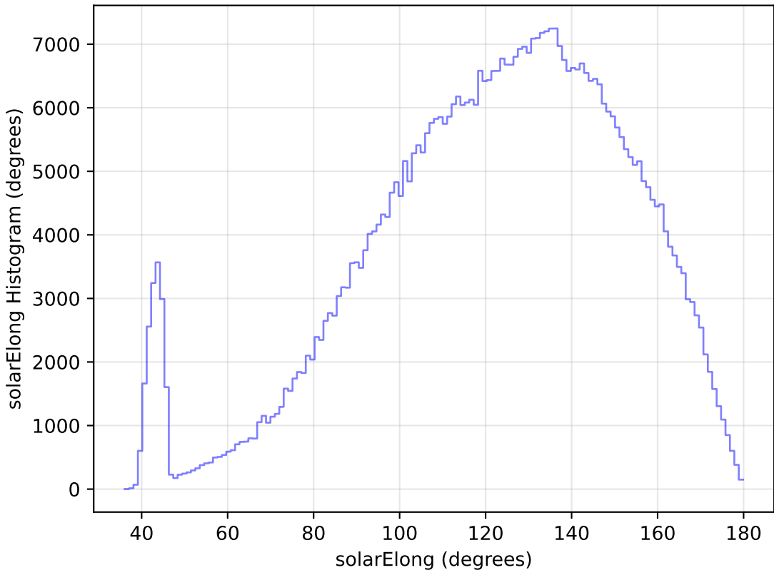
weather_cloudso20v3.4_10yrs WFD r band: solarElong Histogram
