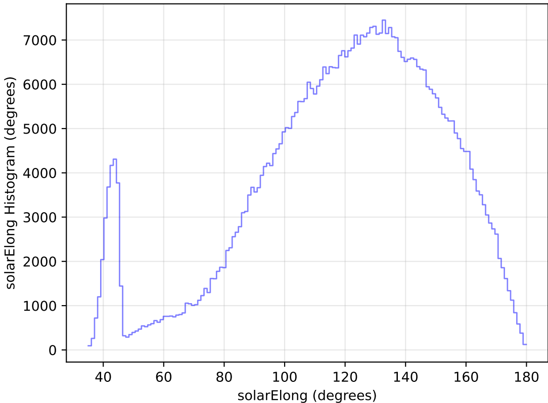
weather_cloudso20v3.4_10yrs WFD i band: solarElong Histogram
