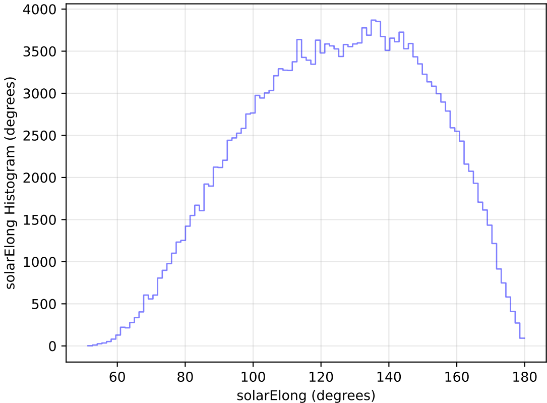
weather_cloudso20v3.4_10yrs WFD g band: solarElong Histogram
