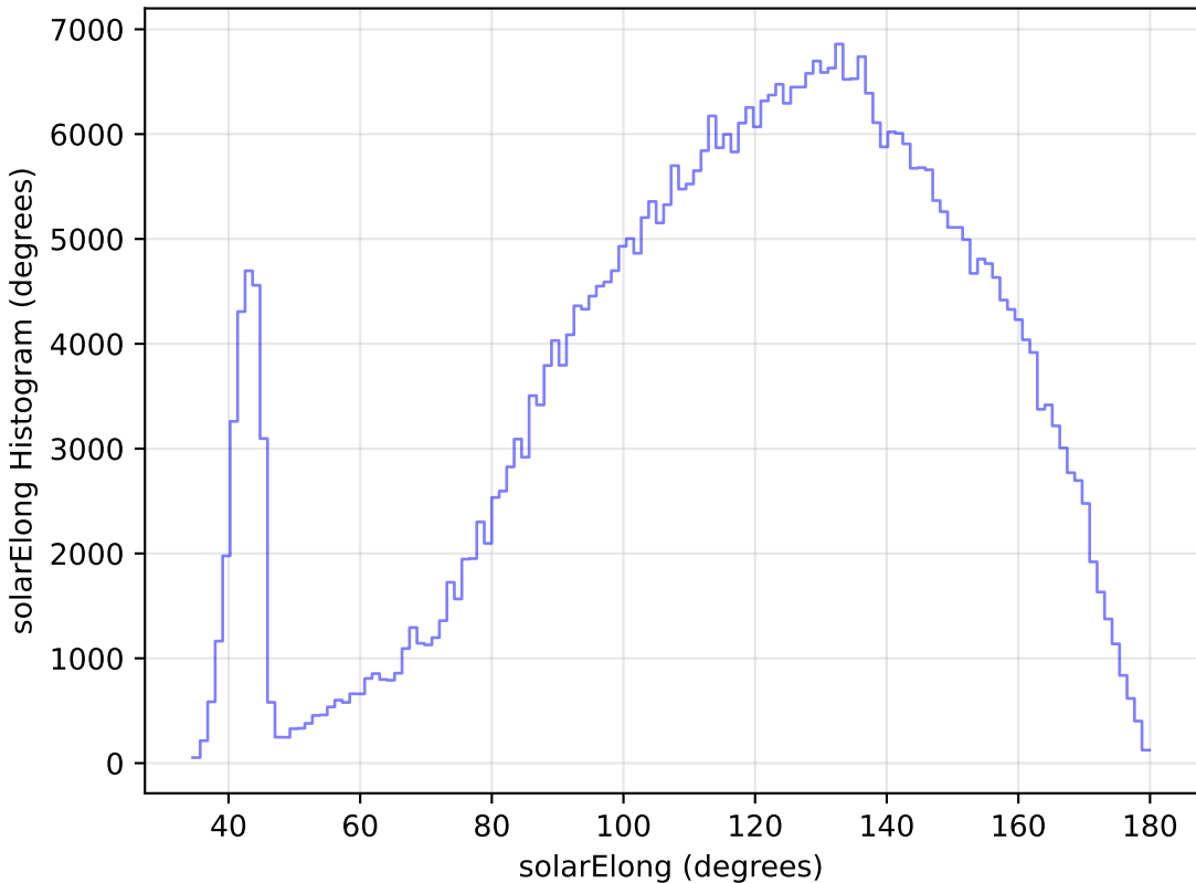
weather_cloudso20v3.4_10yrs All sky z band: solarElong Histogram
