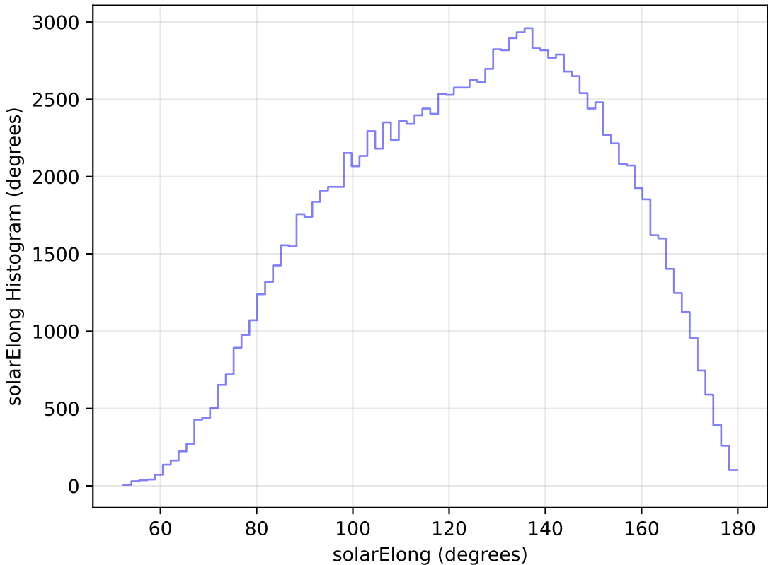
weather_cloudso20v3.4_10yrs All sky u band: solarElong Histogram
