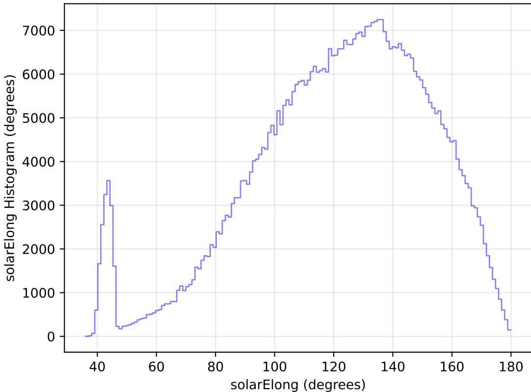
weather_cloudso20v3.4_10yrs All sky r band: solarElong Histogram
