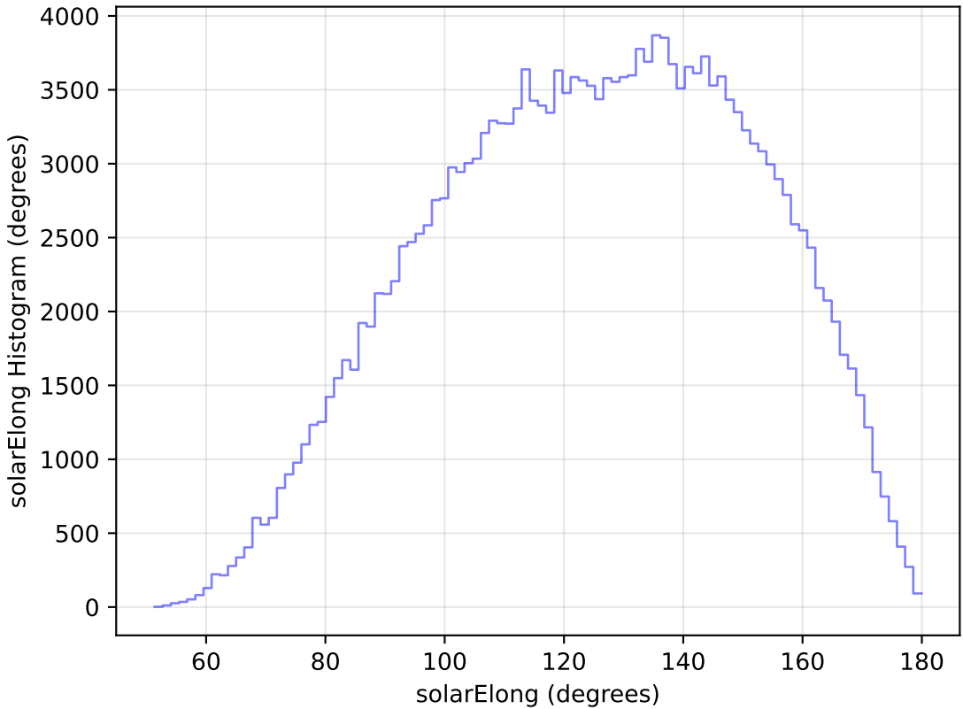
weather_cloudso20v3.4_10yrs All sky g band: solarElong Histogram
