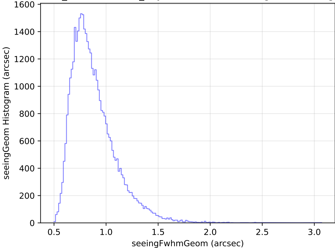
weather_cloudso20v3.4_10yrs Yr 1 z band: seeingGeom Histogram
