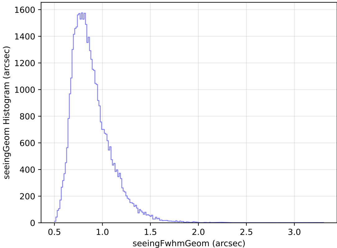
weather_cloudso20v3.4_10yrs Yr 1 y band: seeingGeom Histogram
