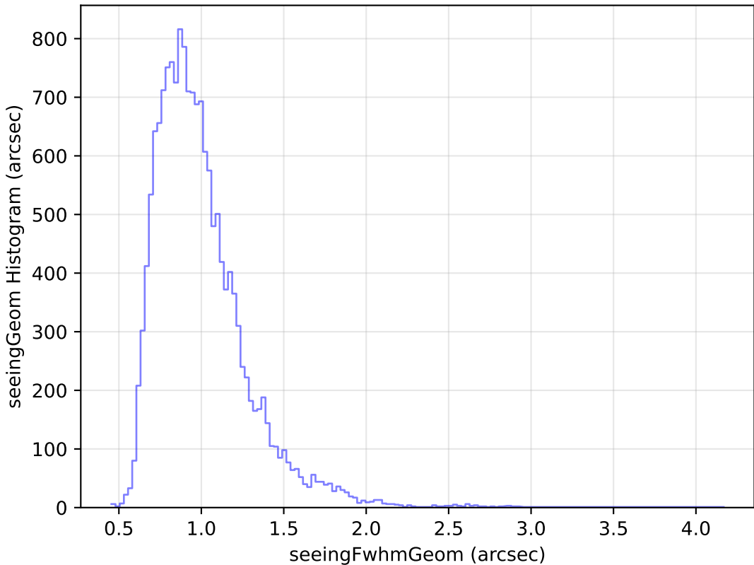
weather_cloudso20v3.4_10yrs Yr 1 u band: seeingGeom Histogram
