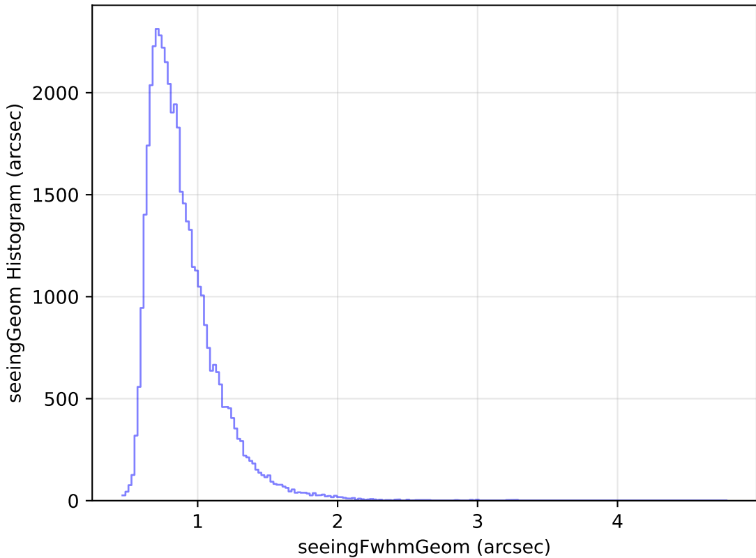
weather_cloudso20v3.4_10yrs Yr 1 r band: seeingGeom Histogram
