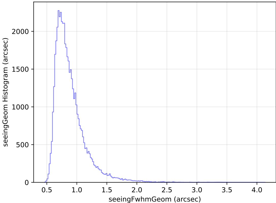
weather_cloudso20v3.4_10yrs Yr 1 i band: seeingGeom Histogram
