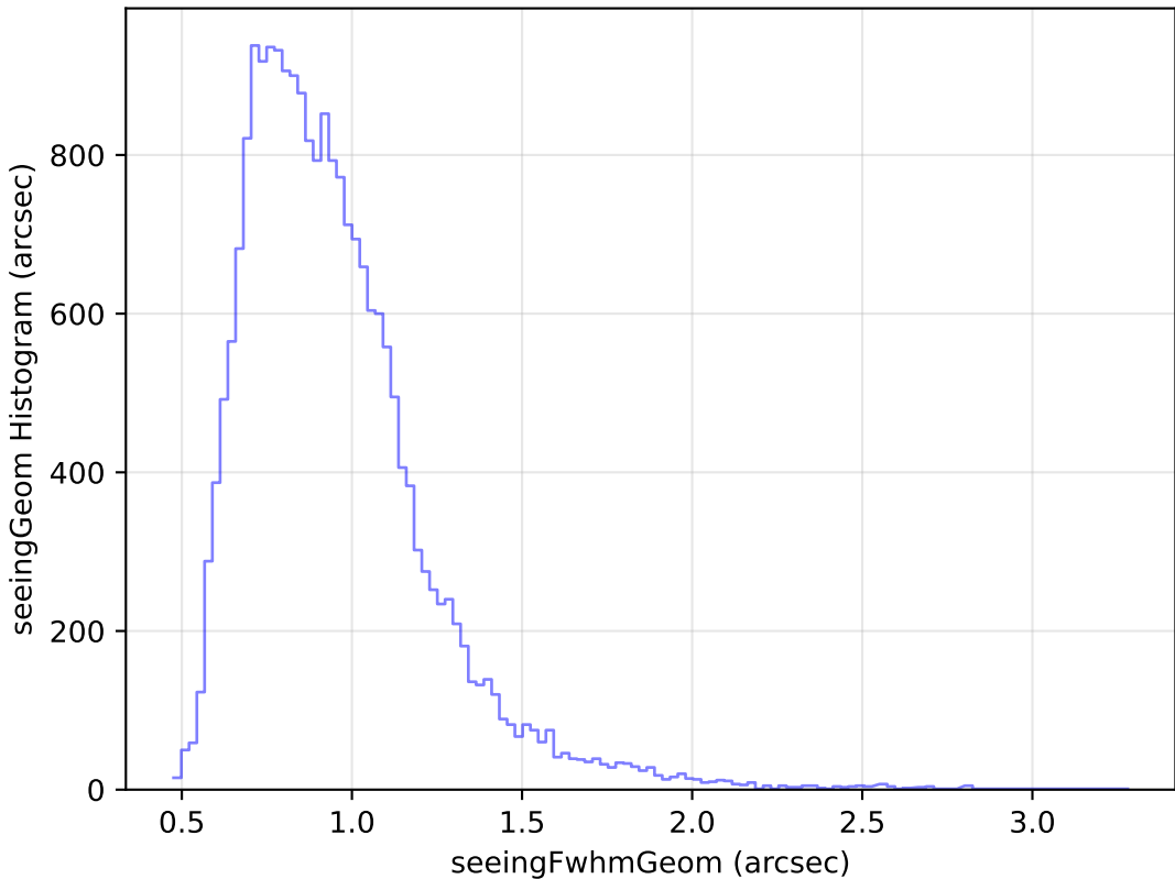
weather_cloudso20v3.4_10yrs Yr 1 g band: seeingGeom Histogram
