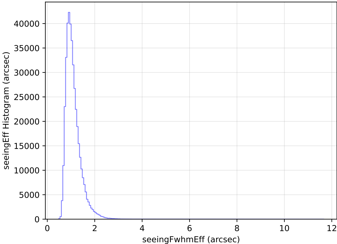
weather_cloudso20v3.4_10yrs WFD y band: seeingEff Histogram
