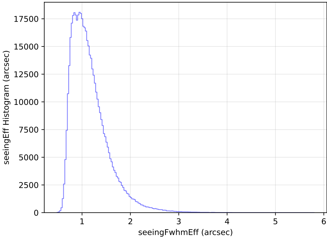
weather_cloudso20v3.4_10yrs WFD r band: seeingEff Histogram
