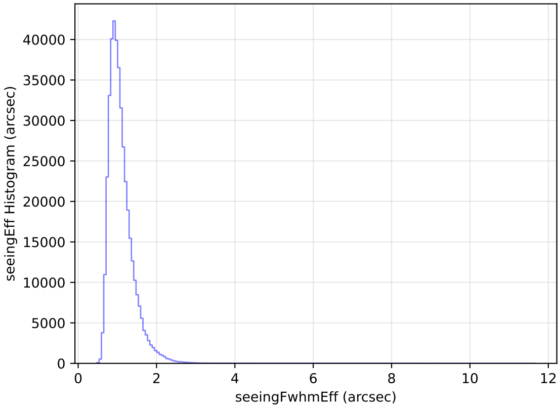
weather_cloudso20v3.4_10yrs All sky y band: seeingEff Histogram
