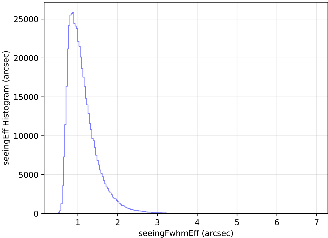
weather_cloudso20v3.4_10yrs All sky i band: seeingEff Histogram
