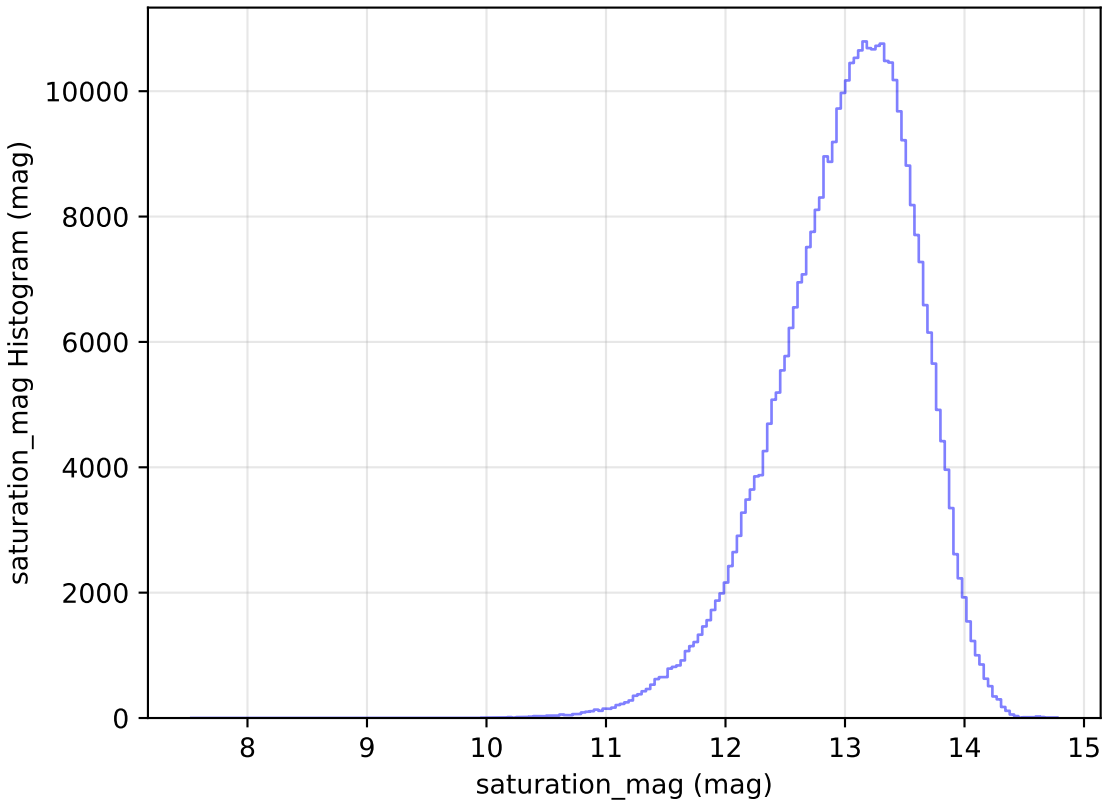
weather_cloudso20v3.4_10yrs WFD y band: saturation_mag Histogram
