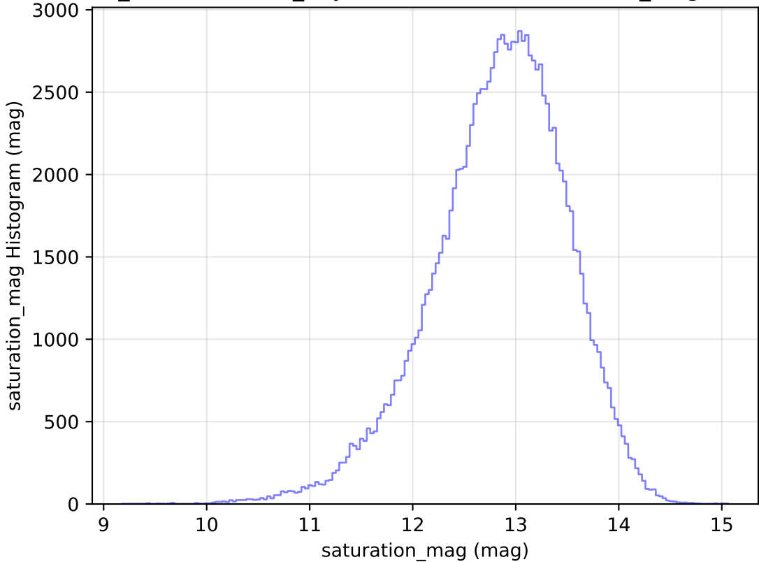
weather_cloudso20v3.4_10yrs WFD u band: saturation_mag Histogram
