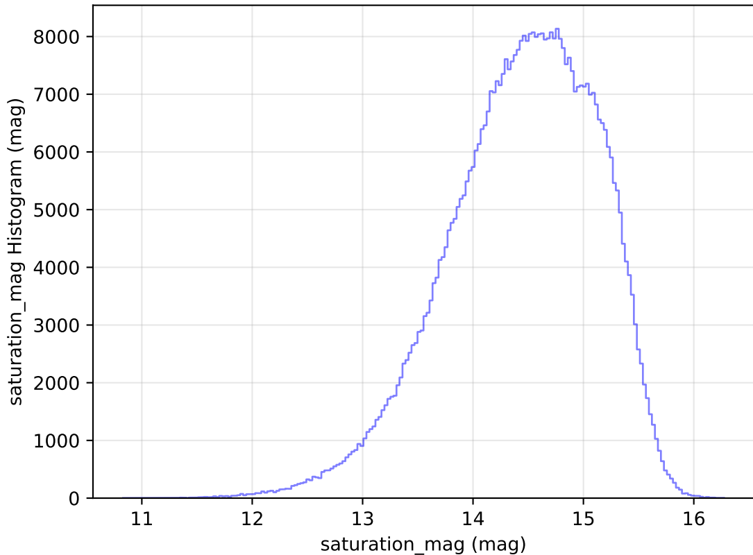
weather_cloudso20v3.4_10yrs WFD r band: saturation_mag Histogram
