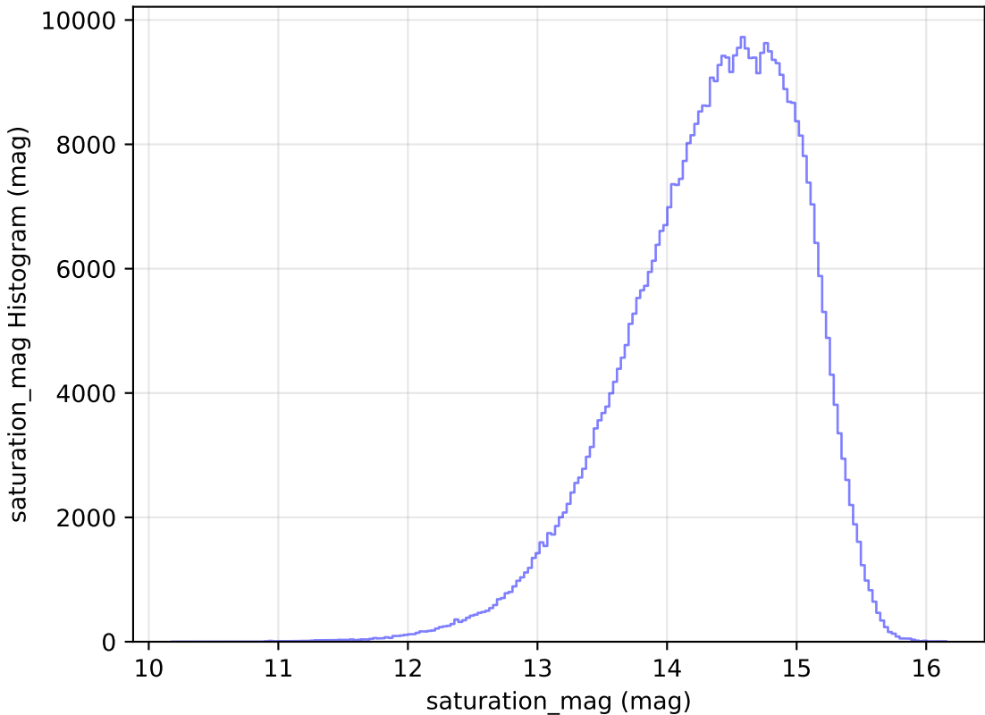
weather_cloudso20v3.4_10yrs WFD i band: saturation_mag Histogram
